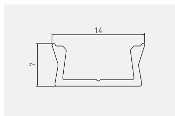
Uchwyt / mounting clip / держатель / кліпса монтажна:
